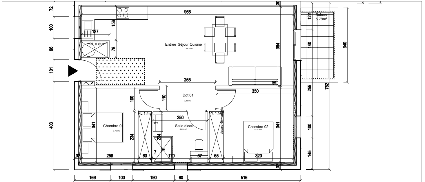
PLAN REZ DE CHAUSSEE Echelle: 1/100 ème BAT N° 11 APPART N° 1111
