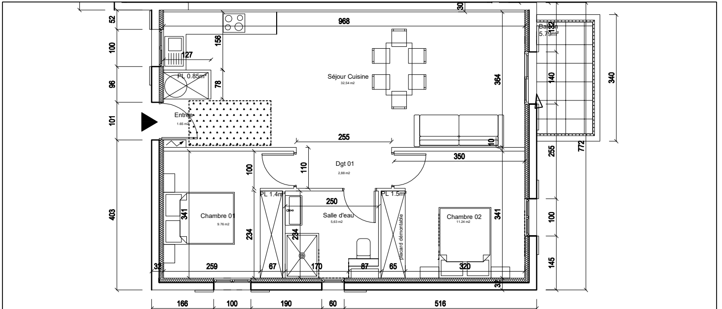
BATIMENT N°03 APPART N°311 PLAN REZ DE CHAUSSEE Echelle: 1/100 ème
