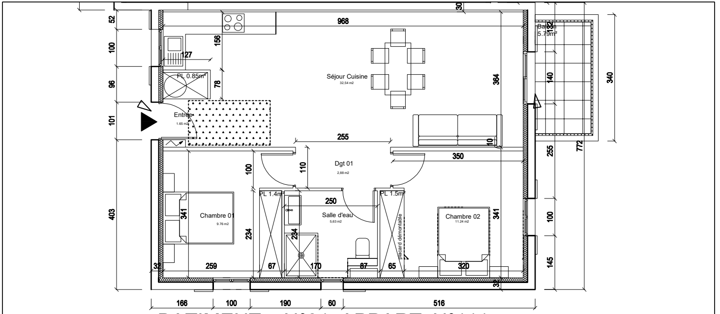
BATIMENT N°01 APPART N°111 PLAN REZ DE CHAUSSEE Echelle: 1/100 ème
