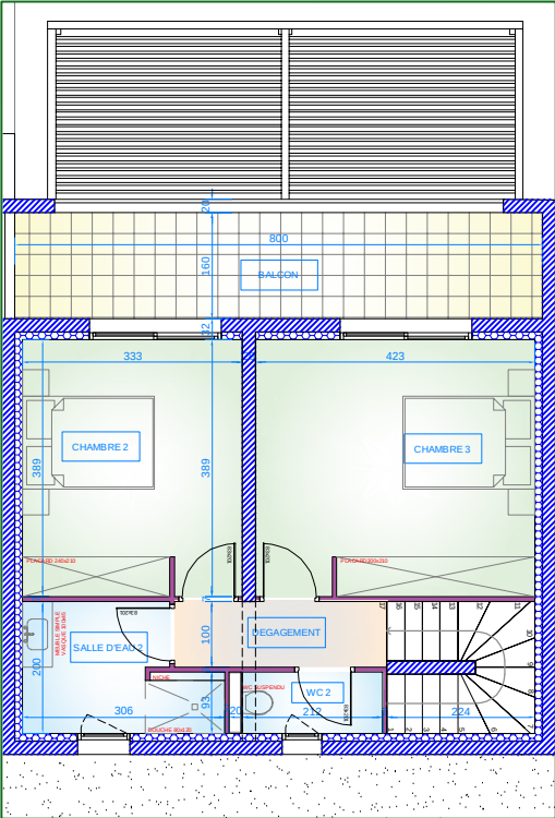
ETAGE
