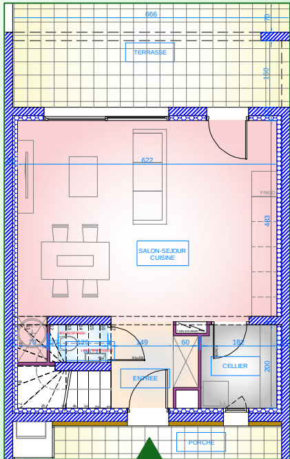
REZ-DE CHAUSSEE
