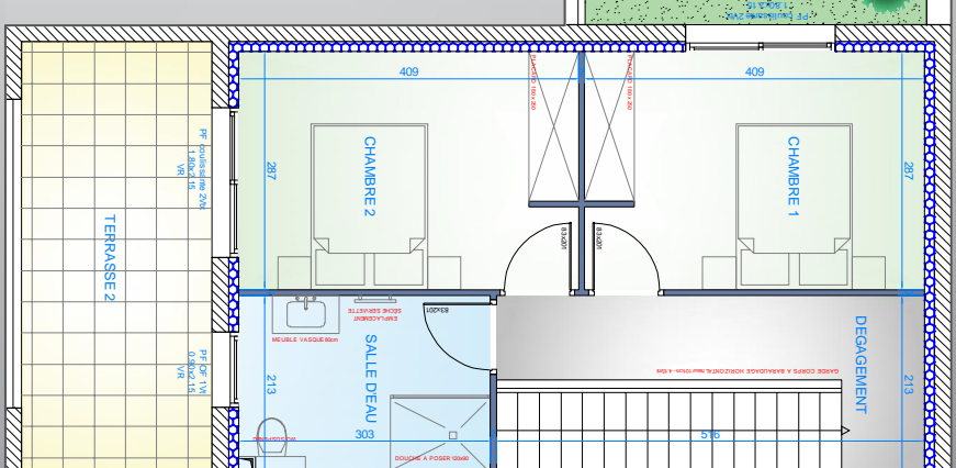
NIVEAU 2 - COIN NUIT
